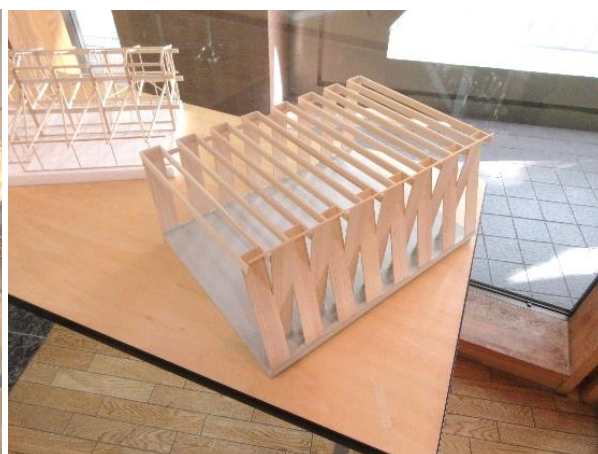
ウトコリミテッド室戸工場 構造模型
